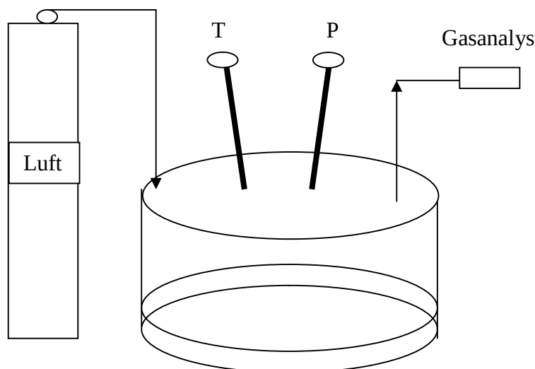
Figur 3. Öppen kammare, exempel. (9)
