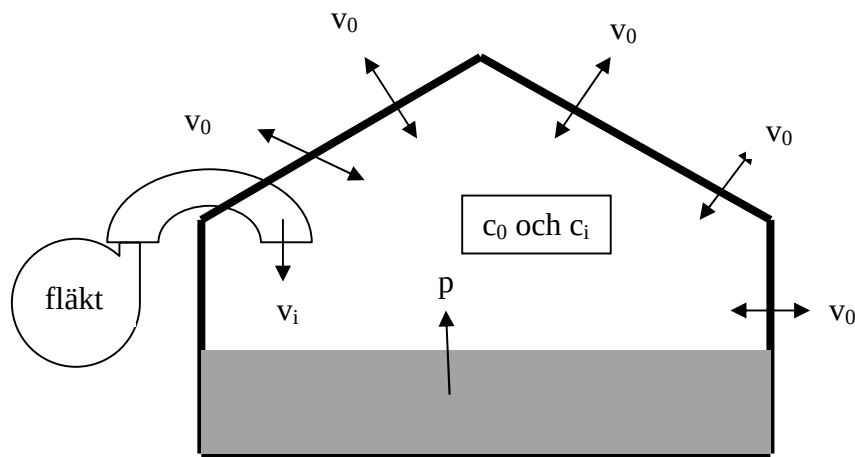
Figur 10. Luftinblåsning i täckt lager, efter (17)
