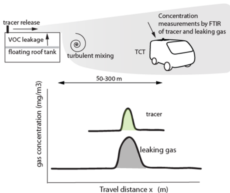
Figur 7. Dynamisk plymmätning, principskiss. Bildkälla: FluxSense
