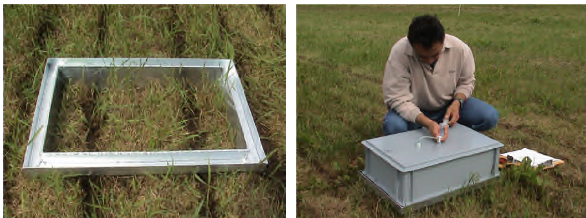
Figur 1. Sluten kammare. Ram med vattenlås till vänster placerad över två gödselsträngar utspridd i vall, provtagning vid förslutning till höger. (7)
