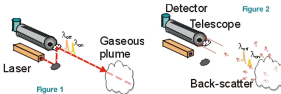
Figur 13. DIAL-tekniken. Bildkälla: www.spectrasyne.ltd.uk
