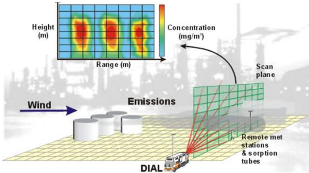
Figur 9. DIAL, principskiss. Bildkälla: www.spectrasyne.ltd.uk
