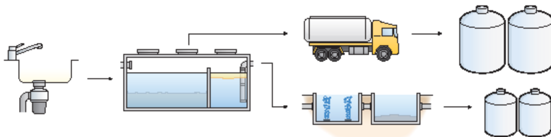
Figur 4 – Systemskiss för insamling, transport och behandling av matavfall som samlats in med köksavfallsbunker till tanksystem. Bild med tillstånd av VA SYD.
